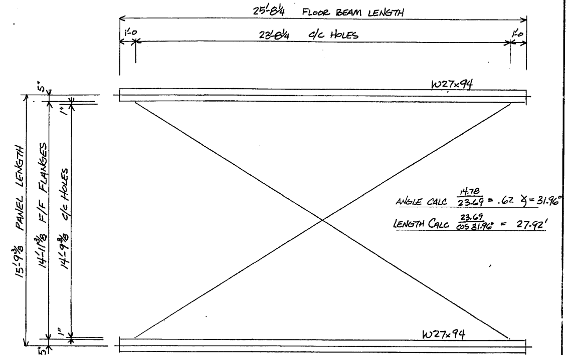
LATERAL ROD LAYOUT
